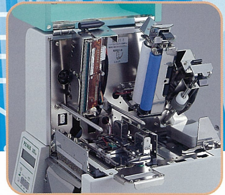
クリーニング機構搭載 搬送路フルオープン
