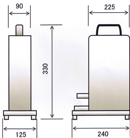
本機概略寸法
